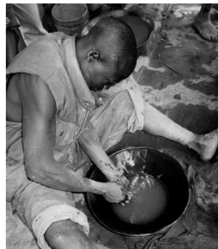
På ytan av kvicksilverbädden anrikas guldstoffet som man samlar upp i en trasa och klämmer ur vattnet så man får en liten kula med guld men där det finns en hel del kvicksilver kvar. För att få fram rent guld ångas kvicksilvret bort under hög värme, "kokas" en farlig process som ofta sker på annan plats av specialister.
